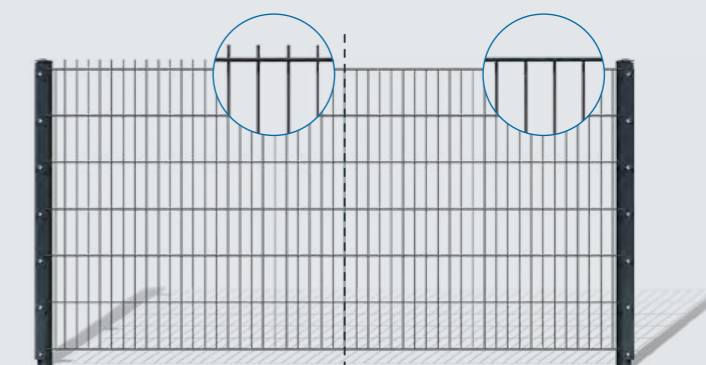
Doppelstabmatte mit Drahtüberstand / ohne Drahtüberstand
